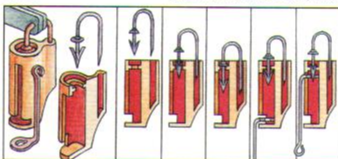
Схема отпираания и запираания.
